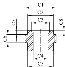
figura G.13 Raccordo filettato M20 × 1,5 Dimensioni in millimetri
