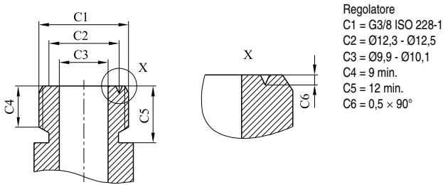
figura H.2 Raccordo filettato 3/8 ISO 228-1 Dimensioni in millimetri
