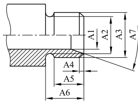
figura G.20 Raccordo filettato 1/4 ISO 228-sinistro Dimensioni in millimetri
