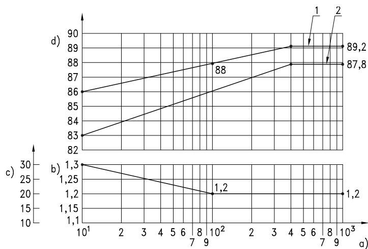
figura 5 Requisiti per le caldaie con camera di combustione in depressione (vedere 5.5)
