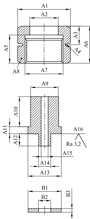
figura G.5 Raccordo filettato 21,8 × 1,814 sin. - 55° - Serraggio con chiave
