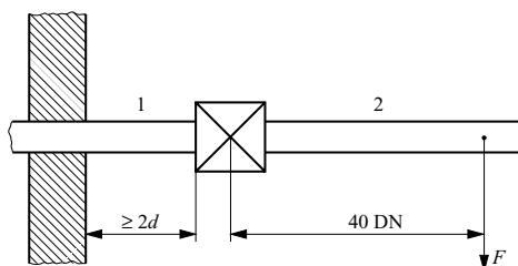
figura 2 Disposizione per la prova di flessione
