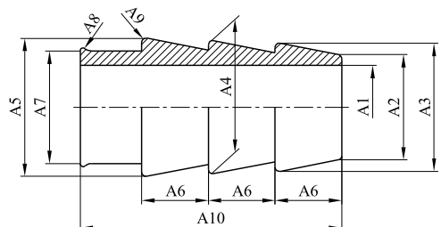
figura H.51 Portagomma - Diametro 10 Dimensioni in millimetri
