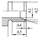
figura G.20 Raccordo filettato 1/4 ISO 228-sinistro Dimensioni in millimetri
