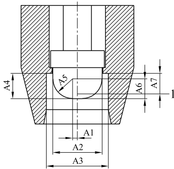
figura G.57 Connessione rapida per rubinetto filettato 21,7 Legenda 1 Riferimento Dimensioni in millimetri Regolatore
