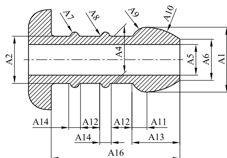
figura H.53 Portagomma - Diametro 8 - 29 Dimensioni in millimetri
