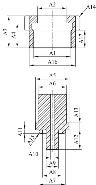
figura G.12 Raccordo filettato 21,8 × 1,814 - 55° sinistro - Serraggio manuale Dimensioni in millimetri
