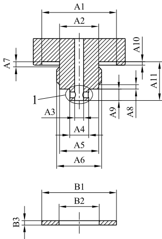
figura G.3 Raccordo filettato M16 × 1,5 destro Legenda 1 Esempio Dimensioni in millimetri Regolatore
