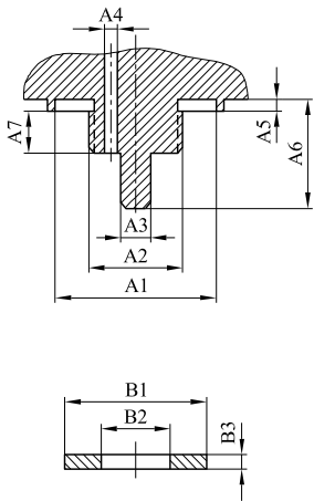
figura G.21 Raccordo filettato Rp 14,8 × 1/18 ISO 7 Regolatore
