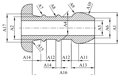
figura H.52 Portagomma - Diametro 13 - 48 Dimensioni in millimetri
