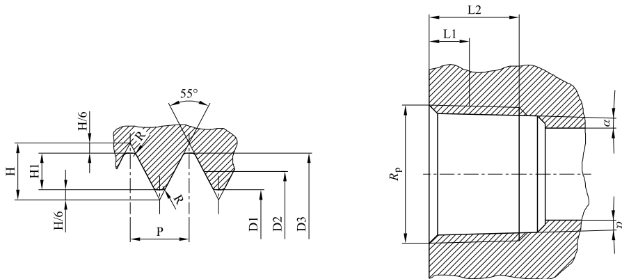
figura H.56 Filettatura interna ISO 7-1 R_c
