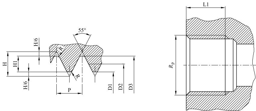
figura H.7 Filettatura interna ISO 7-1
