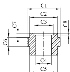
figura H.1 Raccordo filettato M20 × 1,5 Dimensioni in millimetri
