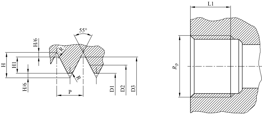
figura G.14 Filettatura interna ISO 7-1 R_p
