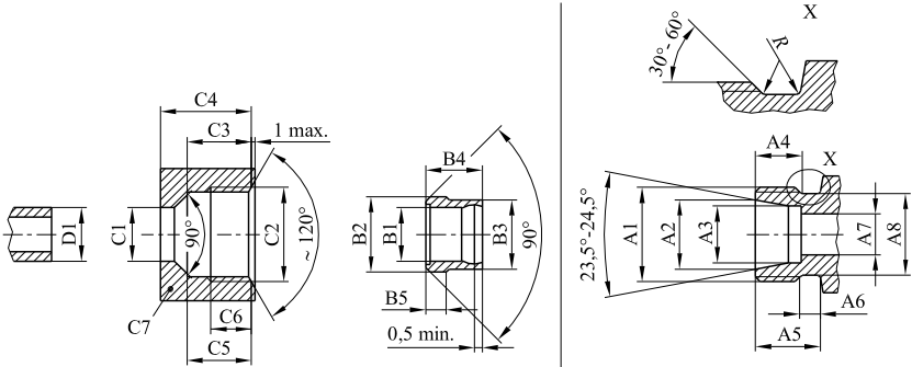
figura G.15 Raccordi a compressione Dimensioni in millimetri Raccordo
