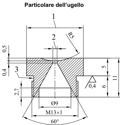
figura6 Prove di funzionamento: Esempio di implementazione del metodo degli ugelli calibrati Legenda 1 Esagonale/Piano 16 2 Diametro alesatura 3 Scarico del fondo filetto Dimensioni in millimetri
