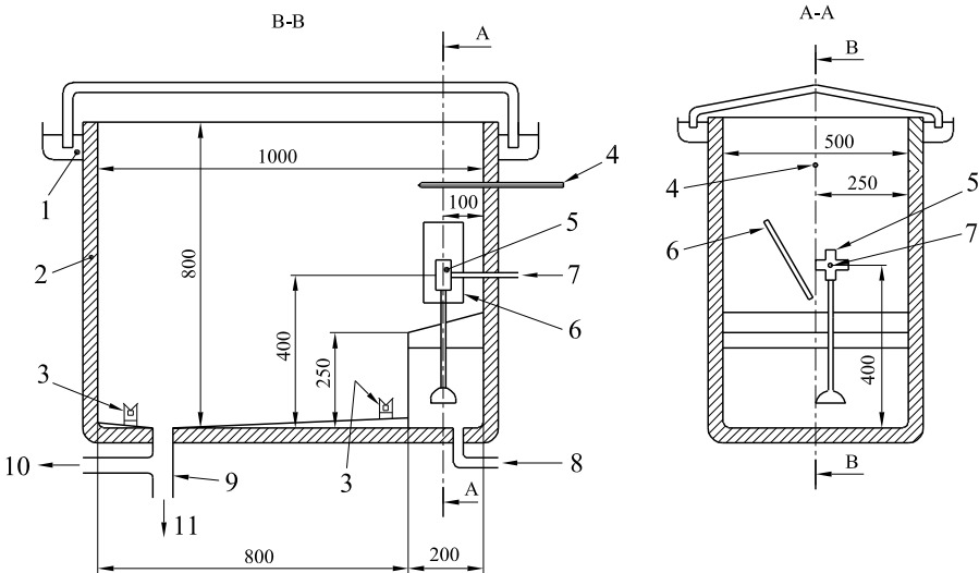
figura L.1 Schema della camera di nebulizzazione Legenda 1 Chiusura a tenuta idraulica 7 Alimentazione aria compressa 2 Pannello di riscaldamento isolato 8 Alimentazione soluzione salina 3 Due dispositivi di raccolta (area orizzontale di 8 000 mm 2 ) 9 Scolo 4 Termometro 10 Aria 5 Ugello di nebulizzazione 11 Acqua 6 Deflettore ad angolo variabile rispetto al nebulizzatore Dimensioni in millimetri
