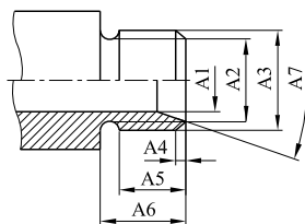
figura H.4 Raccordo filettato - Uscita 1/4 ISO 228 - sinistro Dimensioni in millimetri
