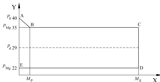
a) Limiti operativi per p_d = 29 mbar butano
