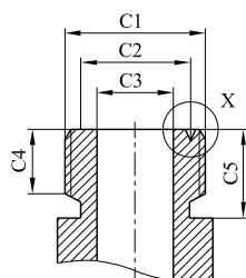
figura H.3 Raccordo filettato 1/2 ISO 228-1 Dimensioni in millimetri
