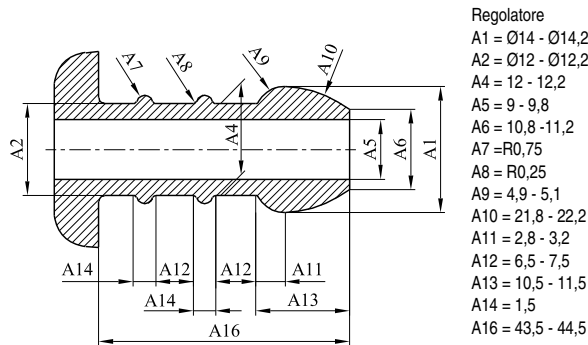
figura H.54 Portagomma - Diametro 13 - 44 Dimensioni in millimetri
