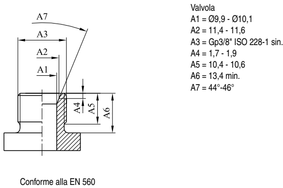
figura H.6 Raccordo filettato - Uscita 3/8 ISO 228 sinistro
