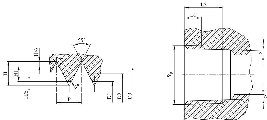
figura G.23 Filettatura interna ISO 7-1 R_c
