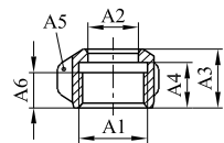
figura G.19 Raccordo filettato 21,8 × 1,814 sinistro ISO 228-1 Dimensioni in millimetri Regolatore
