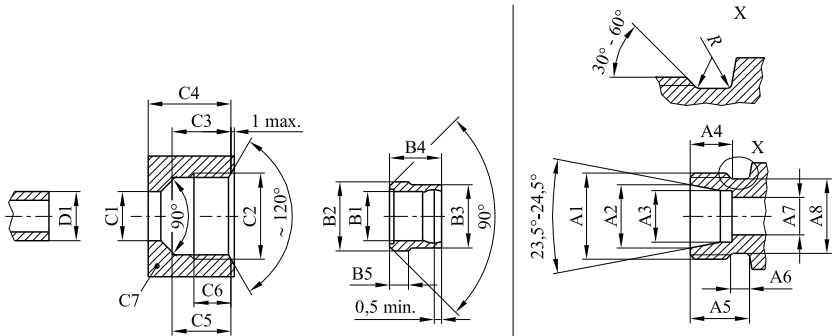
figura H.9 Raccordi a compressione Raccordo
