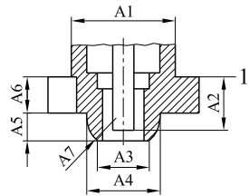
figura G.61 Connessione ad innesto rapido a baionetta Legenda 1 Riferimento Dimensioni in millimetri Regolatore
