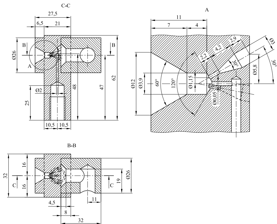
figura L.2 Nebulizzatore di nebbia salina Dimensioni in millimetri
