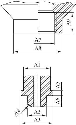
figura G.6 Raccordo filettato 22 × 1,155 sinistro Dimensioni in millimetri Regolatore
