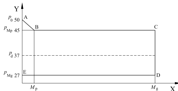
c) Limiti operativi per p_d = 37 mbar propano
