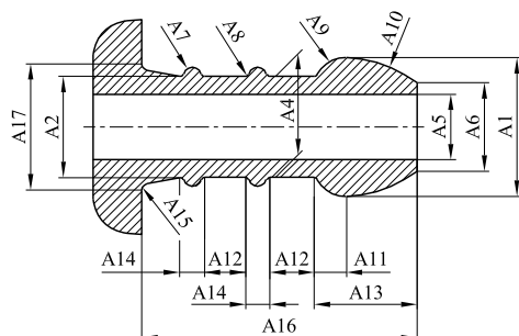
figura H.50 Portagomma - Diametro 8 - 23,5 Dimensioni in millimetri
