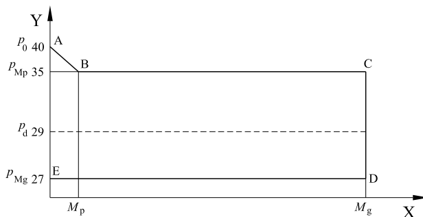
b) Limiti operativi per p_d = 29 mbar GPL
